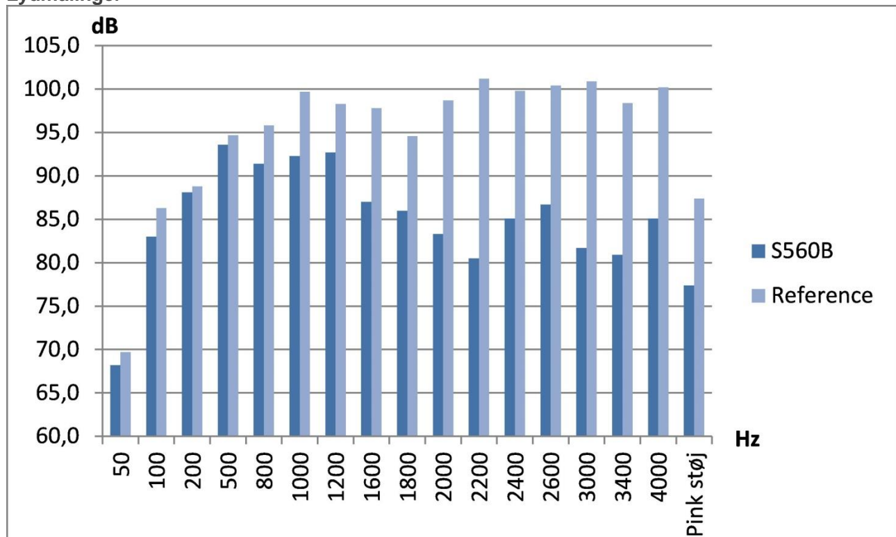
Lydmålinger
